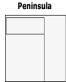
Peninsula LHF 0712/RHF 0711 110cm x 93 x 96cm H LHF 0714/RHF 0713 117cm x 93 x 96cm H LHF 0716/RHF 0715 126cm x 93 x 96cm H LHF 0738/RHF 0737 134cm x 93 x 96cm H
